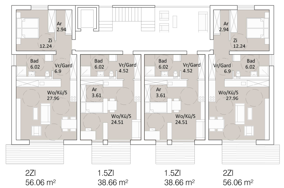
Betreutes Wohnen Regelgeschoß
