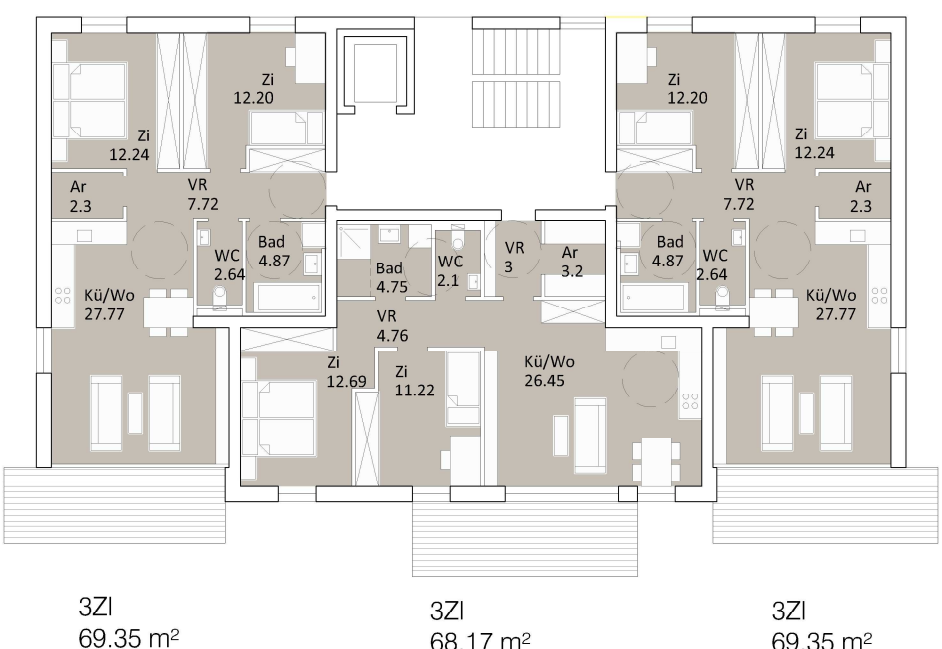
3-Spänner Typ 2 Regelgeschoß (EG-OG3)
