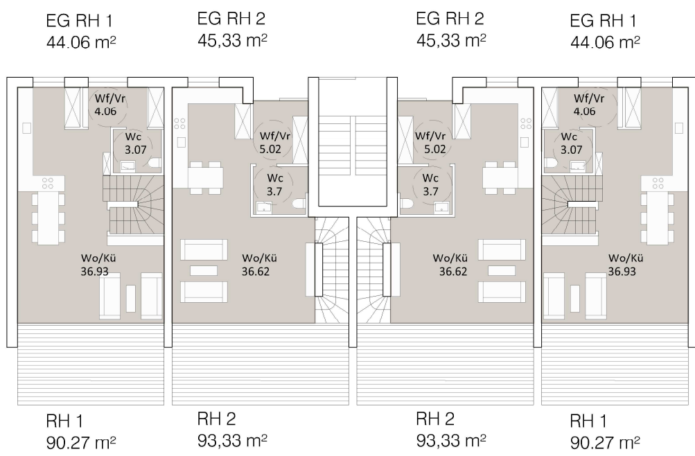
Reihenhaus Erdgeschoß
