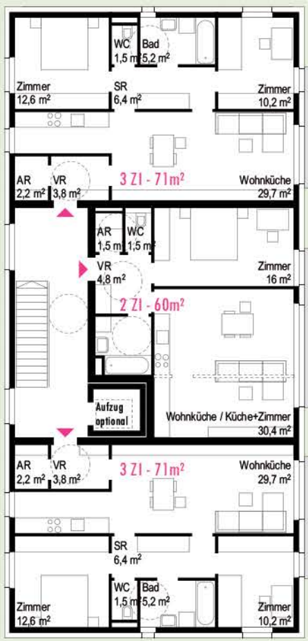
TYP C2 ERDGESCHOSS u. REGELGESCHOSS 2 * 3-Zi zu 71m² 1 * 1-Zi zu 60m²
