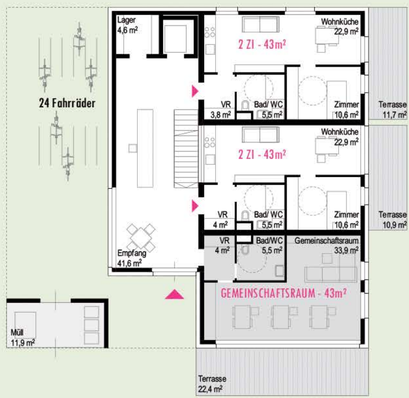
TYP B ERDGESCHOSS GEMEINSCHAFTSRAUM 43m² 2 * 2-Zi zu 43m²
