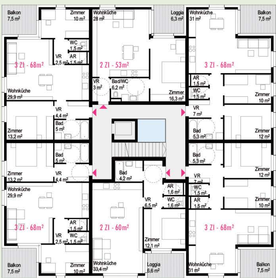
TYP D REGELGESCHOSS 4 * 3-Zi zu 68m² 1 * 2-Zi zu 68m² 1 * 2-Zi zu 53m²
