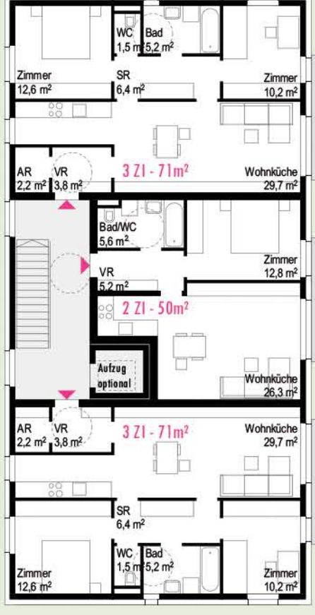
TYP C1 ERDGESCHOSS u. REGELGESCHOSS 2 * 3-Zi zu 71m² 1 * 2-Zi zu 50m²
