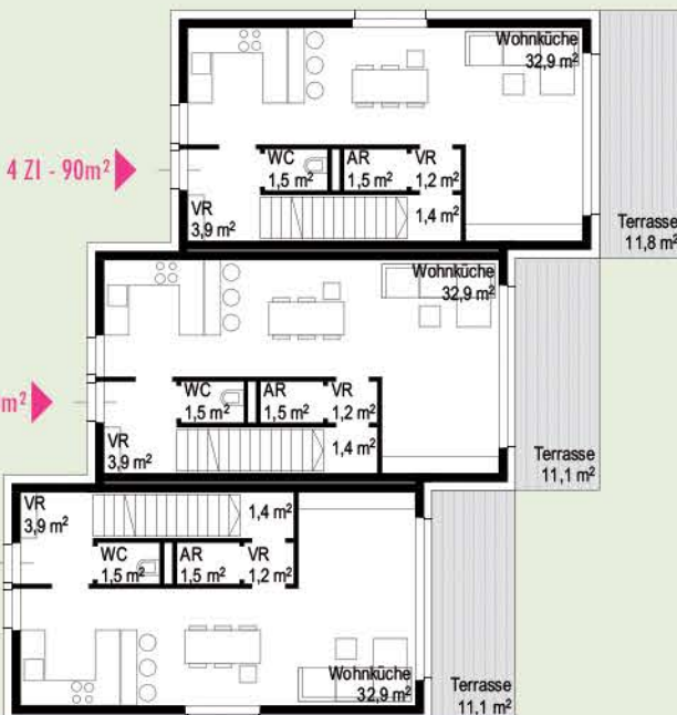
ERDGESCHOSS
